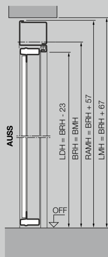
Vertikalschnitt Tür ohne unteren Anschlag
