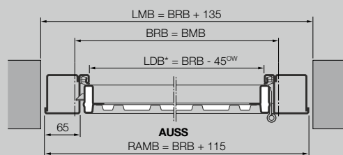
Horizontalschnitt
