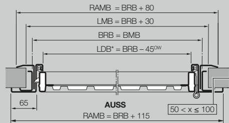
Horizontalschnitt
